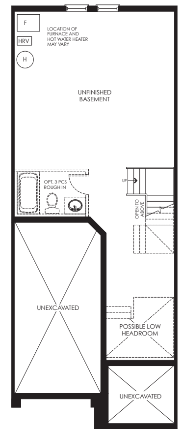
BASEMENT PLAN ELEV. 'A', 'B'
